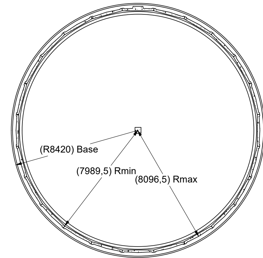
D-D ( 1 : 150 )
