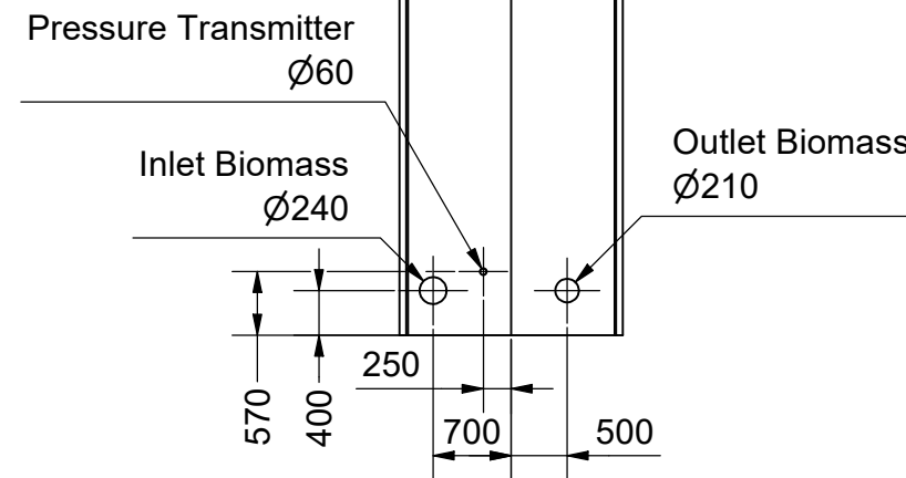
C-C ( 1 : 100 )
