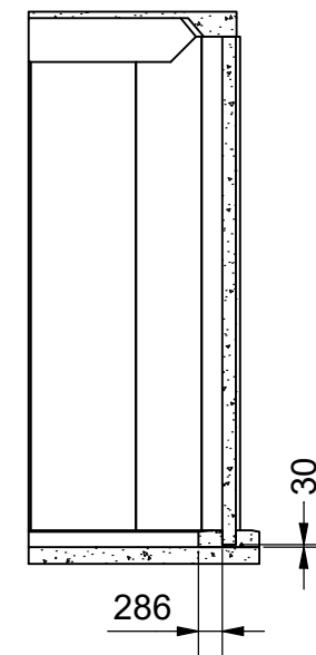
C-C ( 1 : 100 )
